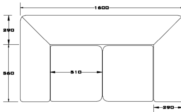
VISTA SUPERIOR
