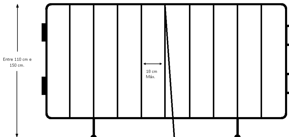
VISÃO FRONTAL
