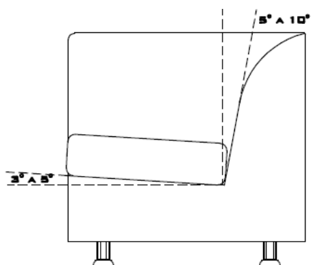
CORTE TRANSVERSAL
