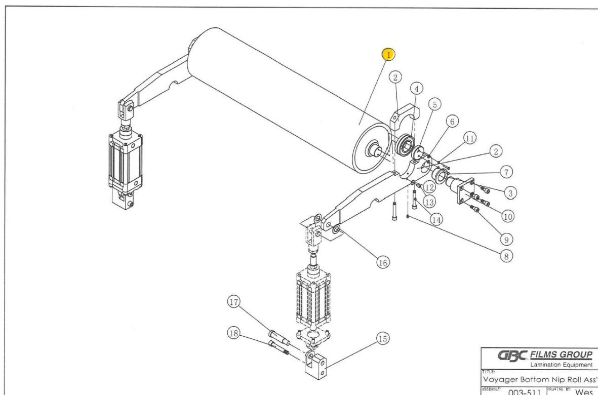
Figura 4 - Esquema de rolo da termolaminadora Mabeg 7580 GBC
