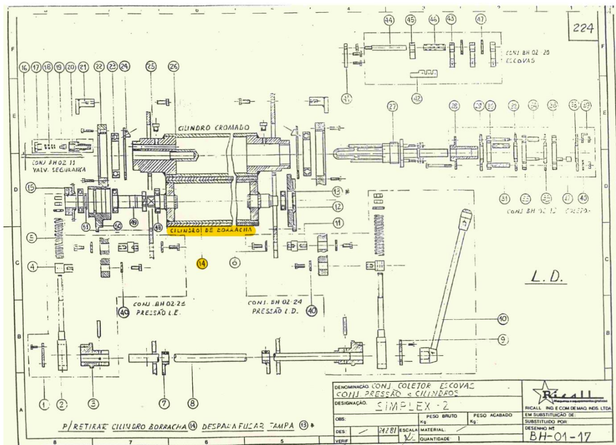
Figura 6 - Esquema de rolo da termolaminadora Ricall Simplex II 82
