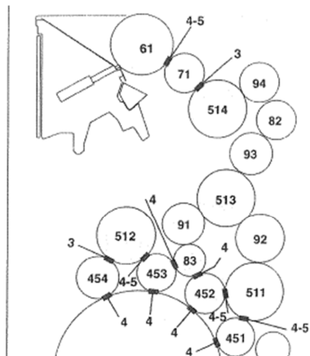
Figura 1 - Esquema de rolos da impressora offset Manroland R708 3B P 4/4
