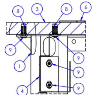
DETALHE B ESCALA 1 : 5
