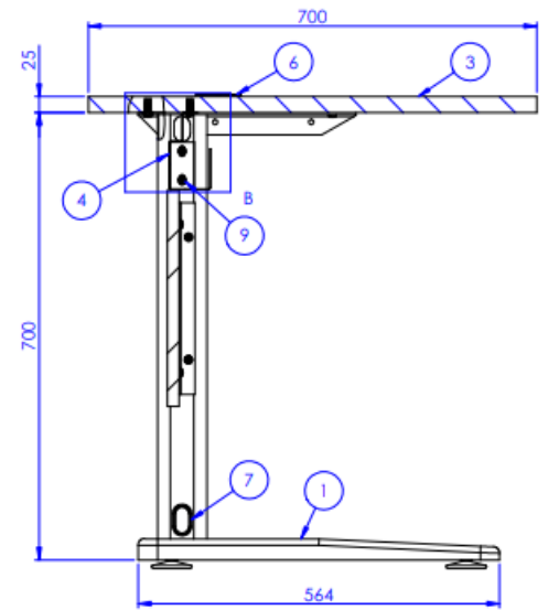
SEÇÃO A-A ESCALA 1 : 13
