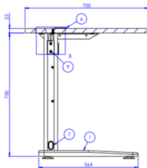
SEÇÃO A-A ESCALA 1 : 13
