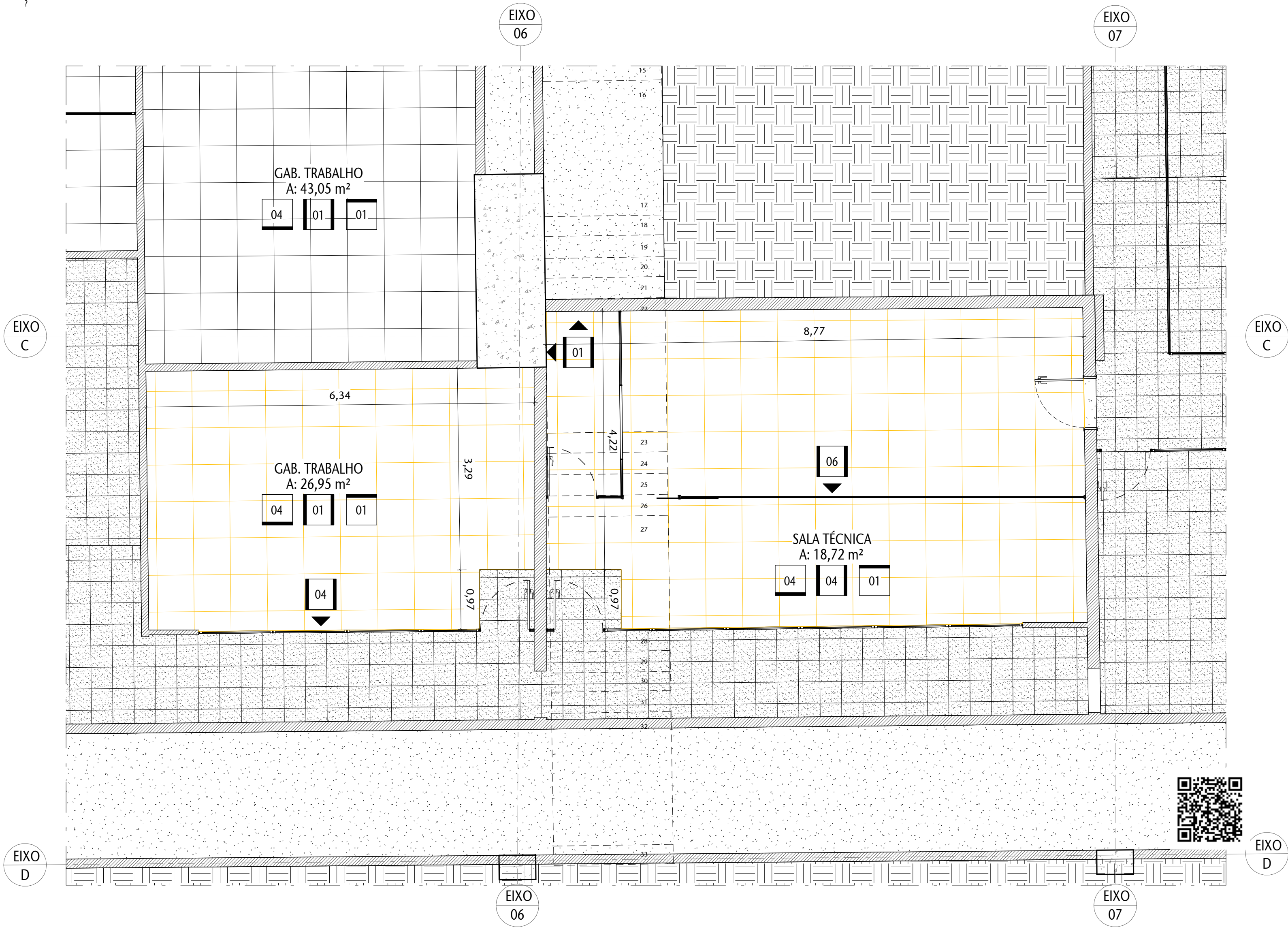
1 PLANTA - DEMOLIR - SUBSOLO - TRECHO 1 ESCALA 1 : 50
