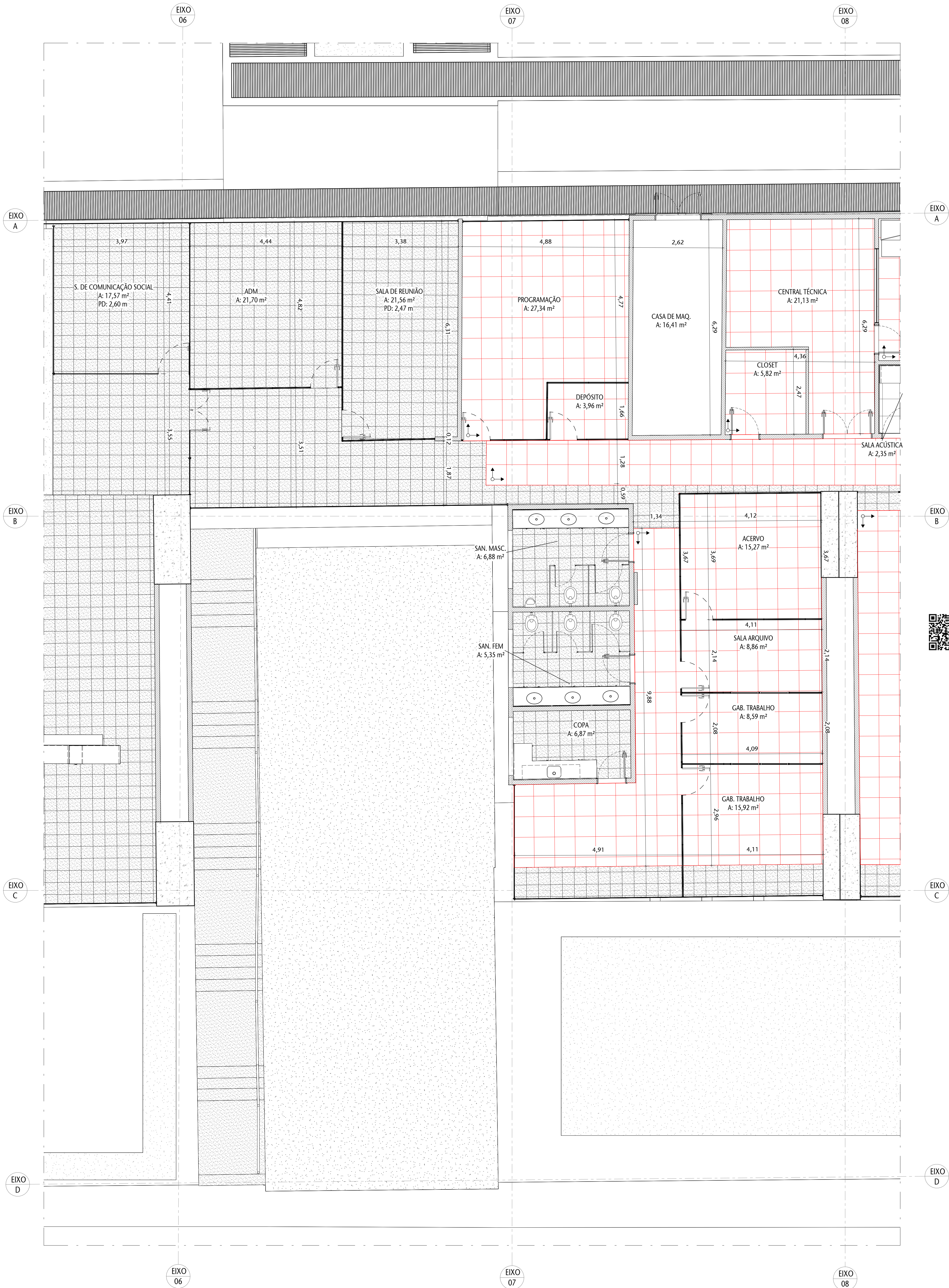
1 PLANTA - CONSTRUIR - TÉRREO - TRECHO 2 ESCALA 1:500
