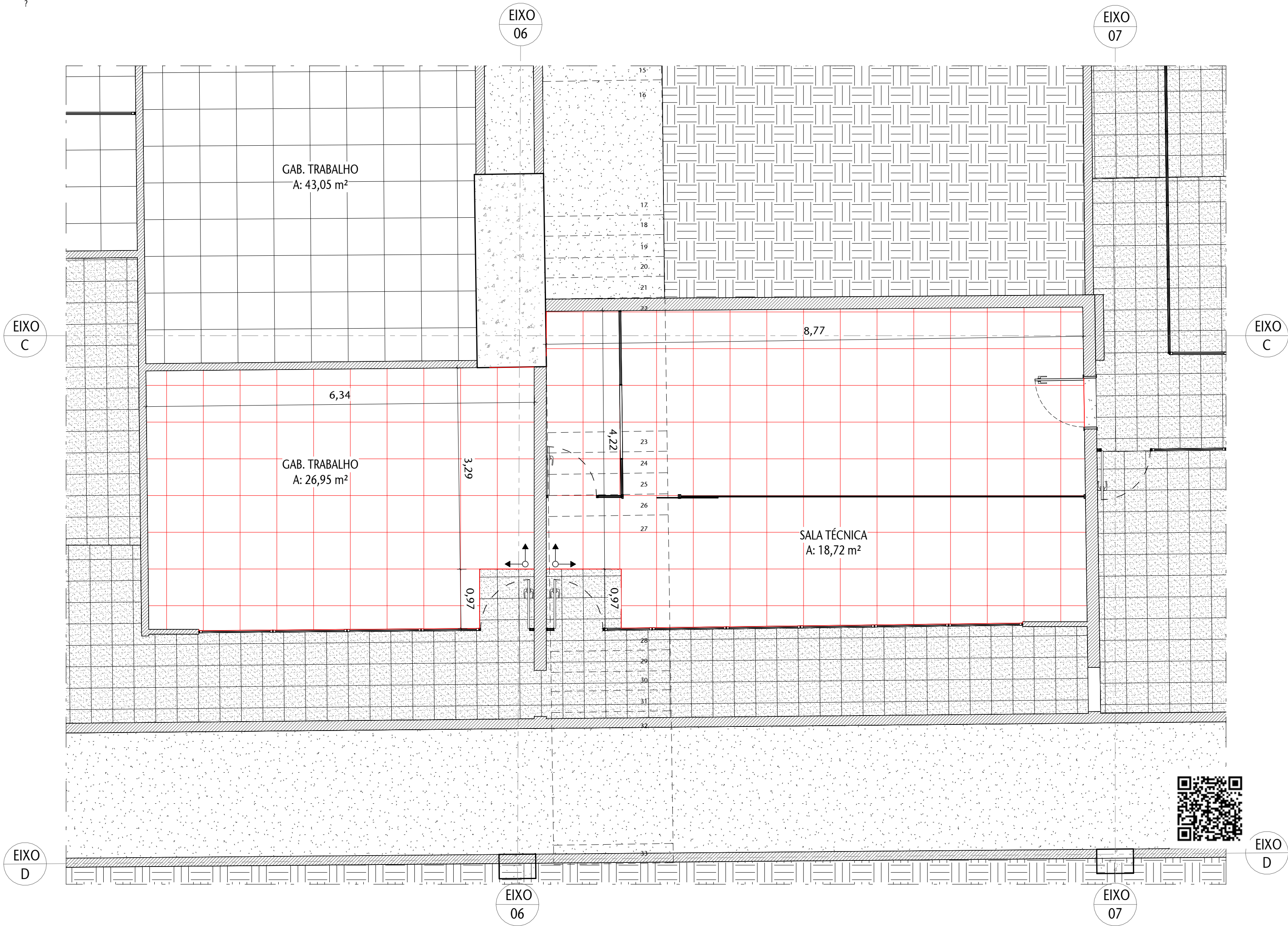
1 PLANTA - CONSTRUIR - SUBSOLO - TRECHO 1 ESCALA 1 : 50
