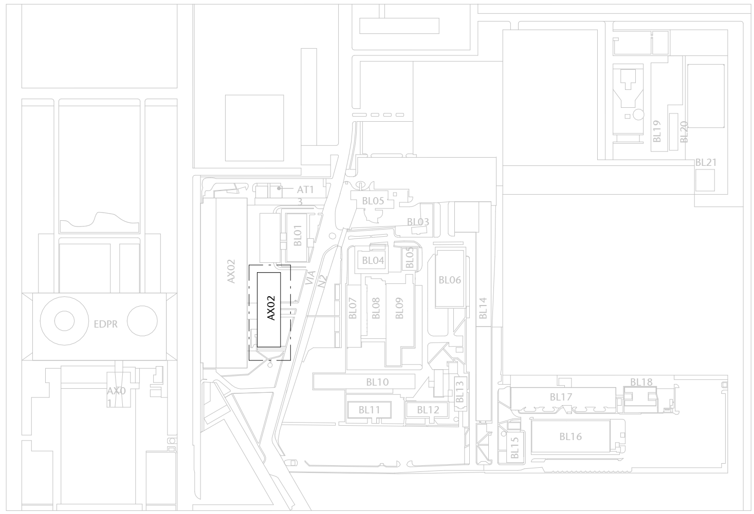
0 PLANTA DE SITUAÇÃO - ANEXO 02 ESCALA 1:1.000
