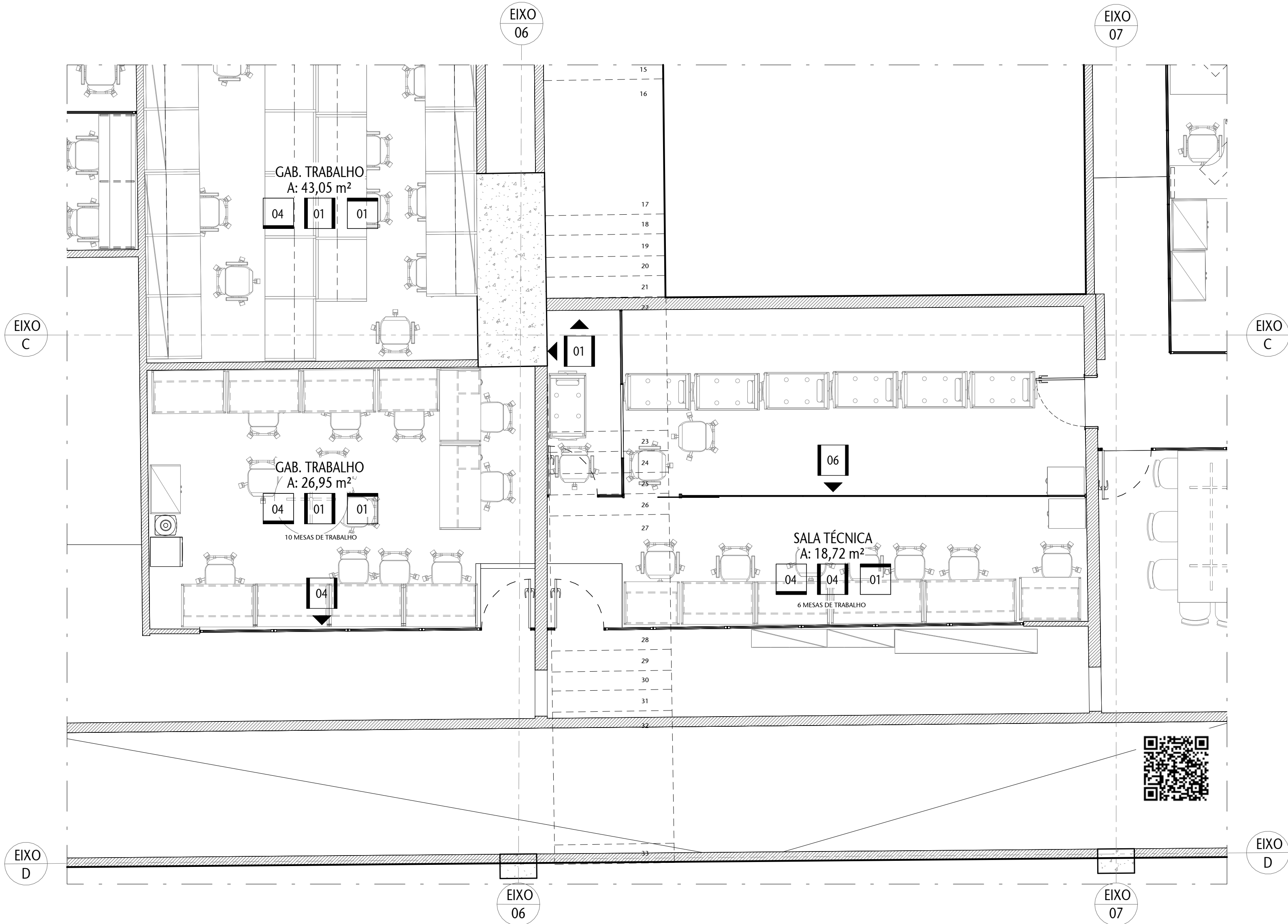
1 PLANTA - LAYOUT COMPLETO - SUBSOLO - TRECHO 1
